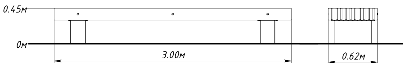
Рисунок 1 — Основные габаритные размеры
