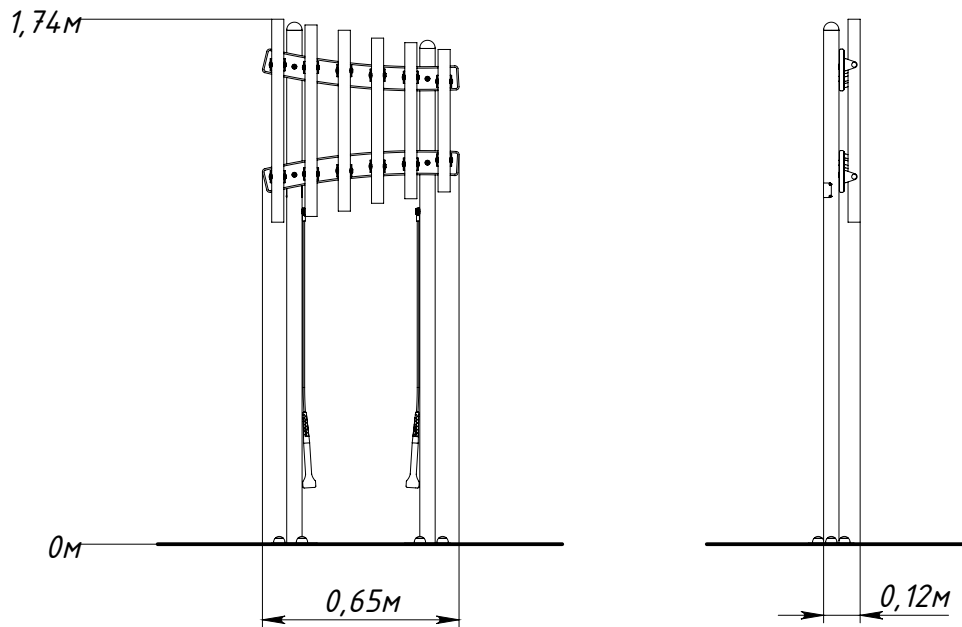
Рисунок 1 — Основные габаритные размеры
