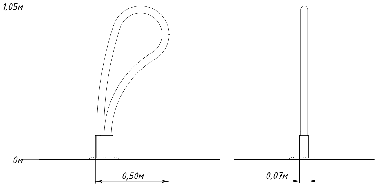
Рисунок 1 — Основные габаритные размеры
