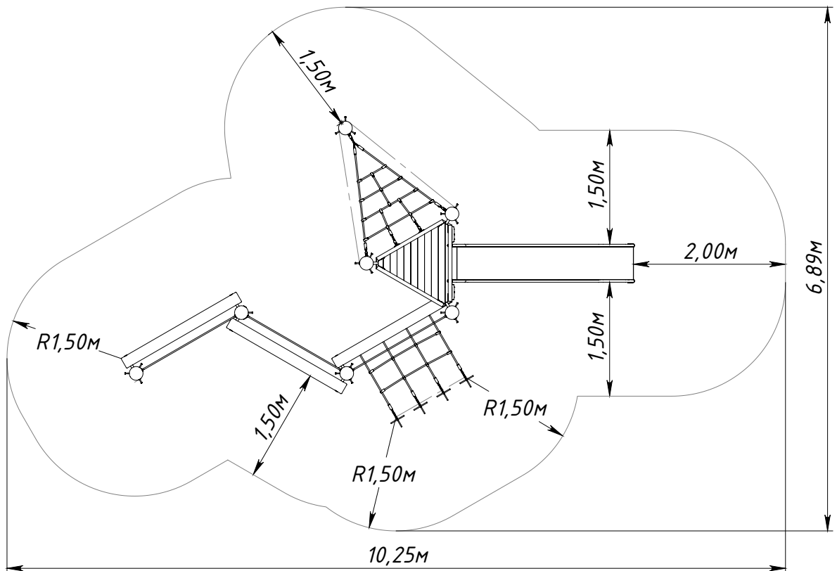
Рисунок 1 — Основные габаритные размеры
