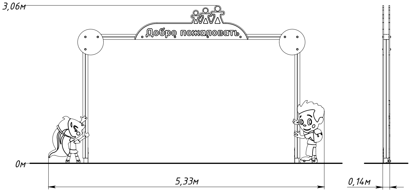
Рисунок 1 — Основные габаритные размеры
