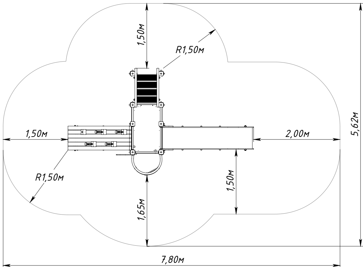
Рисунок 1 — Основные габаритные размеры
