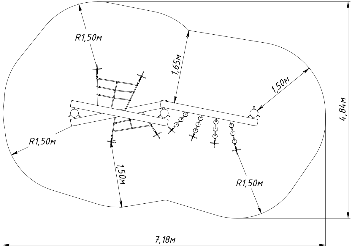
Рисунок 1 — Основные габаритные размеры
