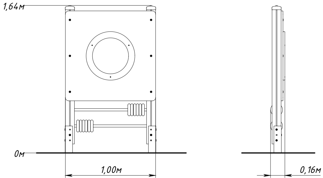
Рисунок 1 — Основные габаритные размеры
