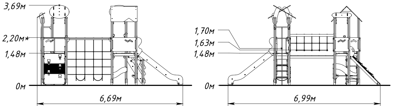
Рисунок 1 — Основные габаритные размеры
