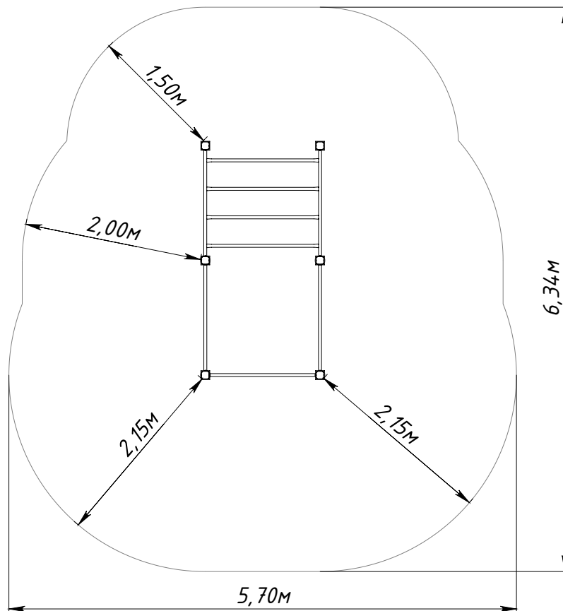
Рисунок 2 — Граница зоны приземления
