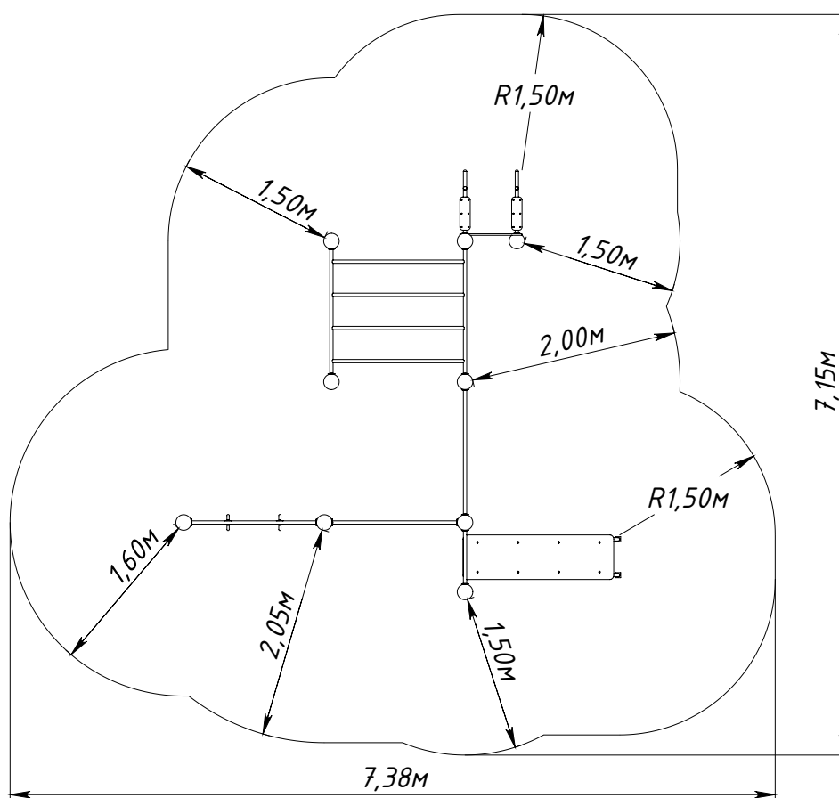
Рисунок 1 — Основные габаритные размеры
