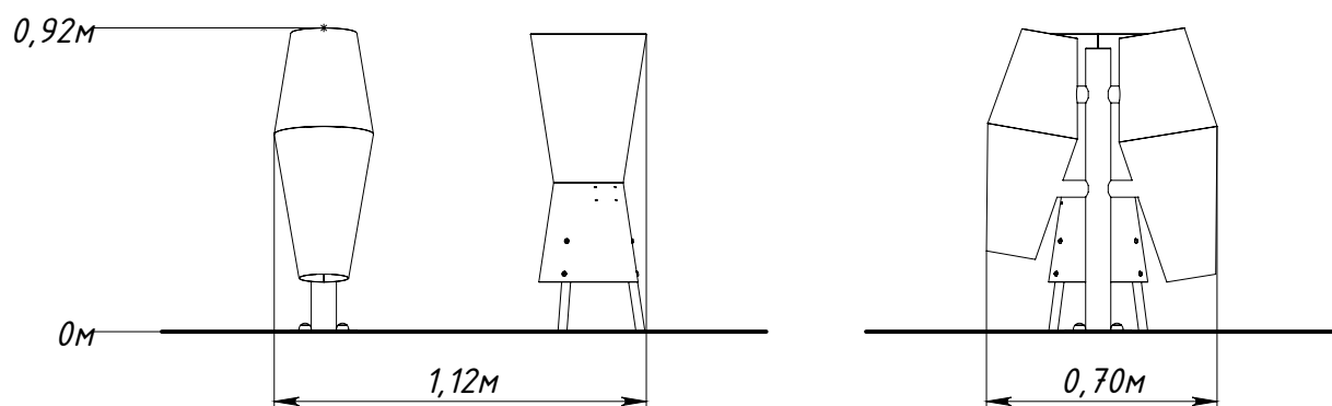
Рисунок 1 — Основные габаритные размеры
