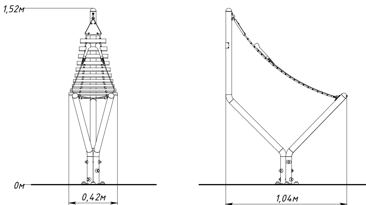
Рисунок 1 — Основные габаритные размеры
