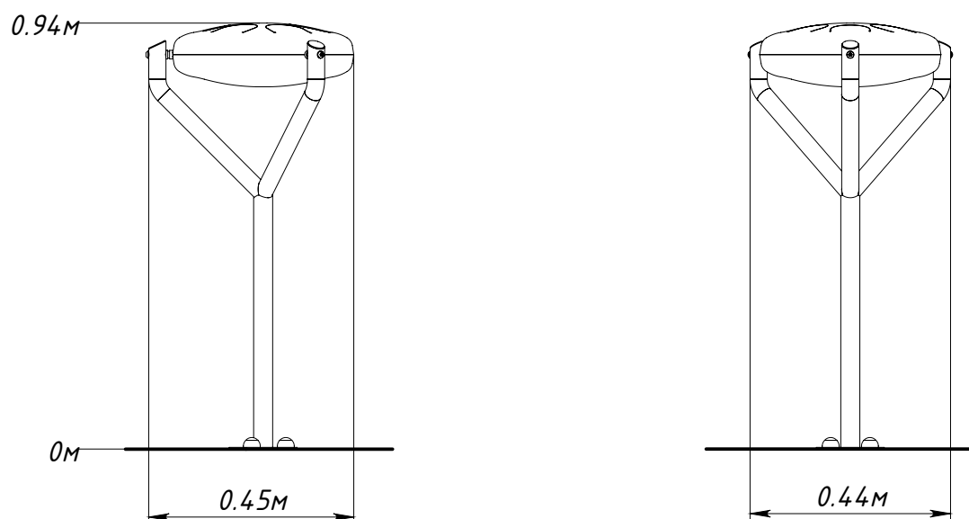
Рисунок 1 — Основные габаритные размеры
