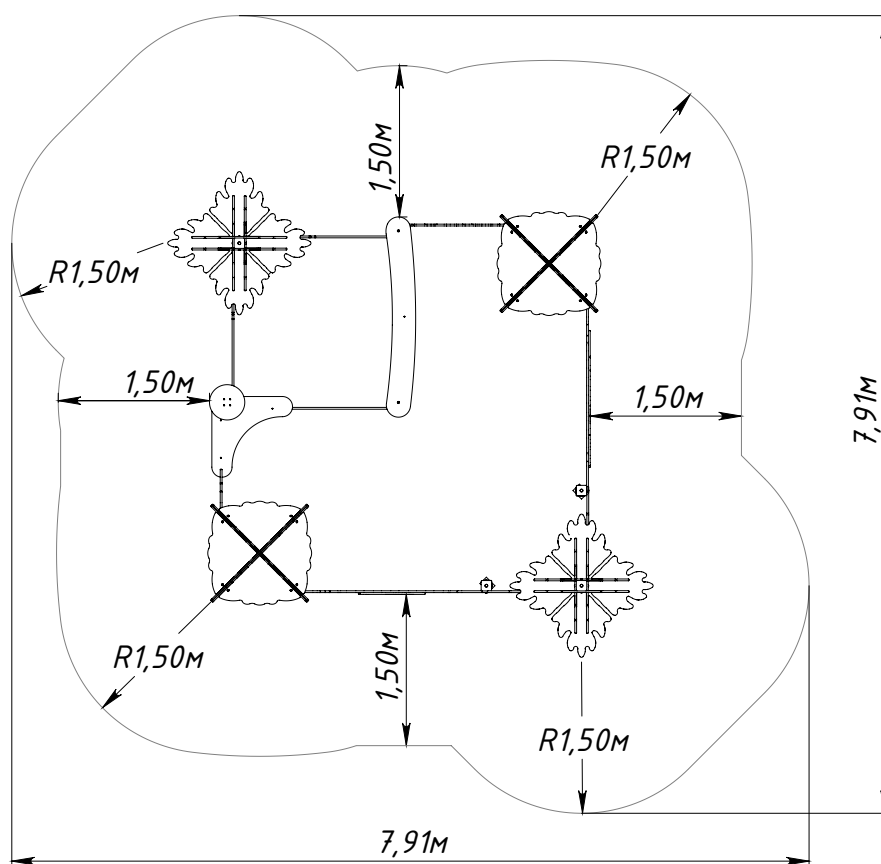
Рисунок 2 — Граница зоны приземления
