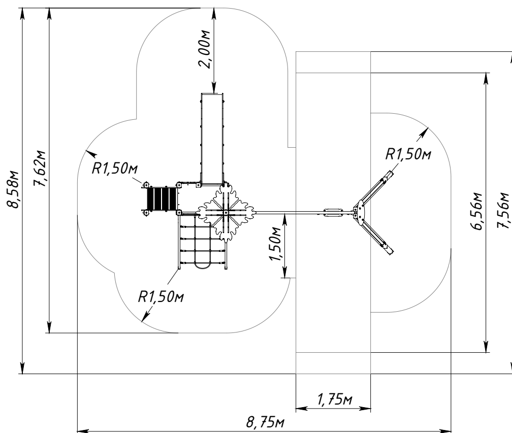
Рисунок 1 — Основные габаритные размеры
