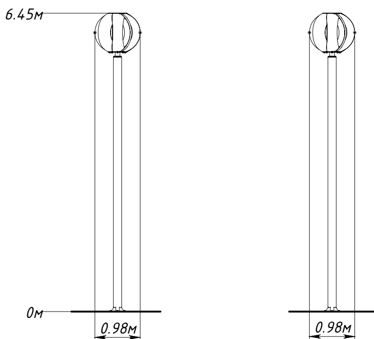
Рисунок 1 — Основные габаритные размеры
