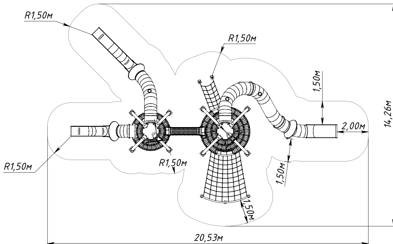
Рисунок 1 — Основные габаритные размеры
