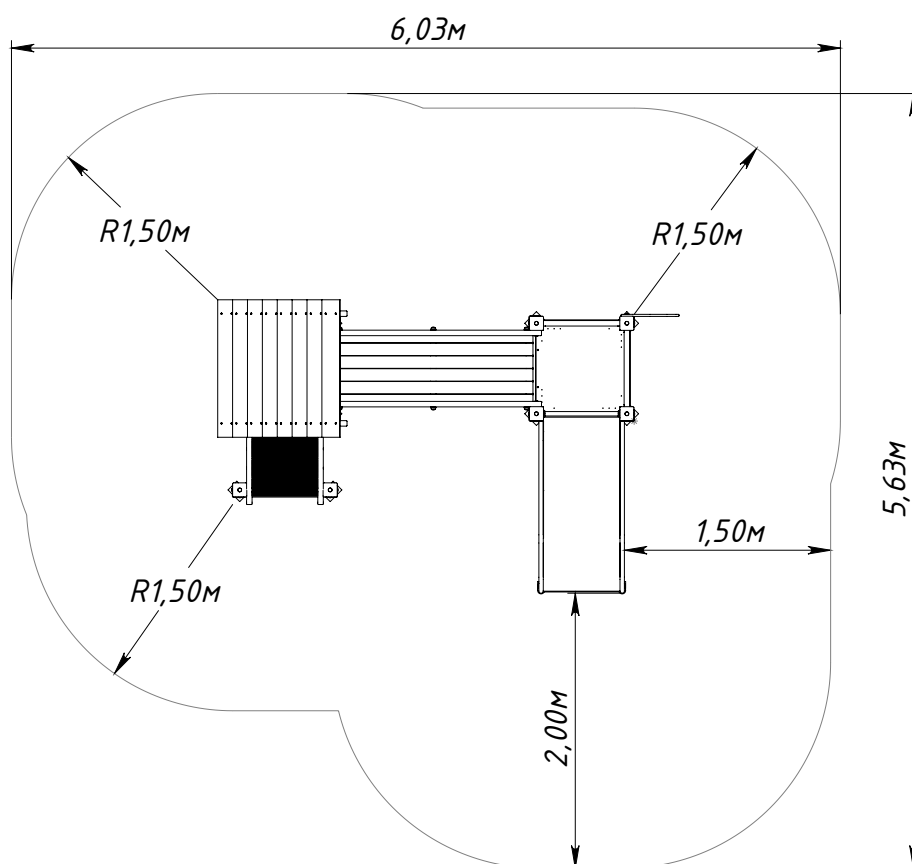
Рисунок 1 — Основные габаритные размеры
