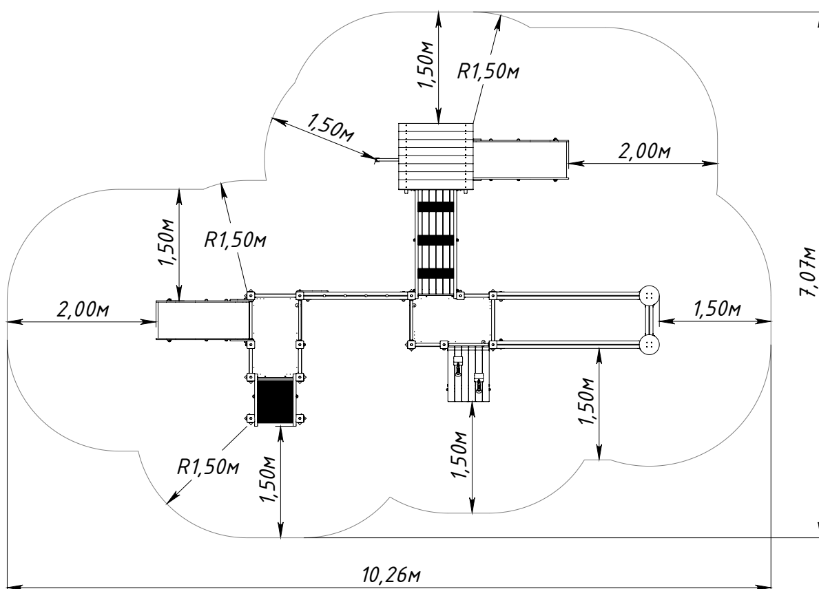
Рисунок 1 — Основные габаритные размеры
