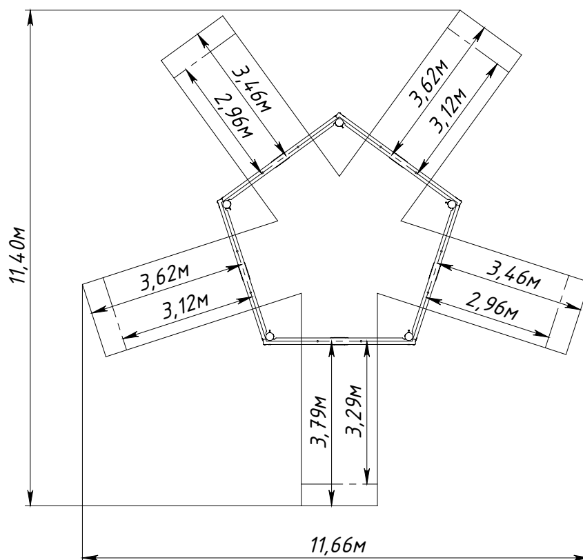
Рисунок 2 — Граница зоны приземления
