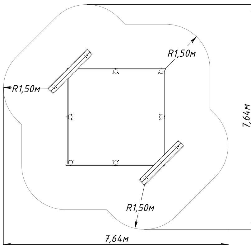
Рисунок 1 — Основные габаритные размеры
