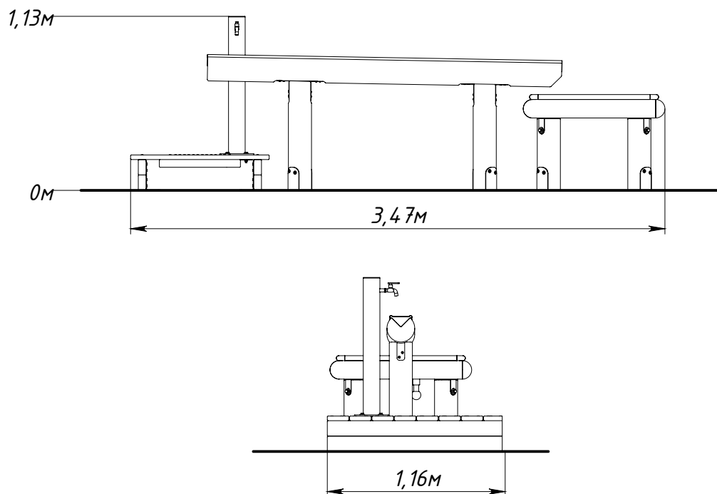
Рисунок 1 — Основные габаритные размеры
