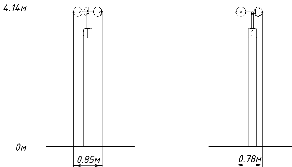
Рисунок 1 — Основные габаритные размеры
