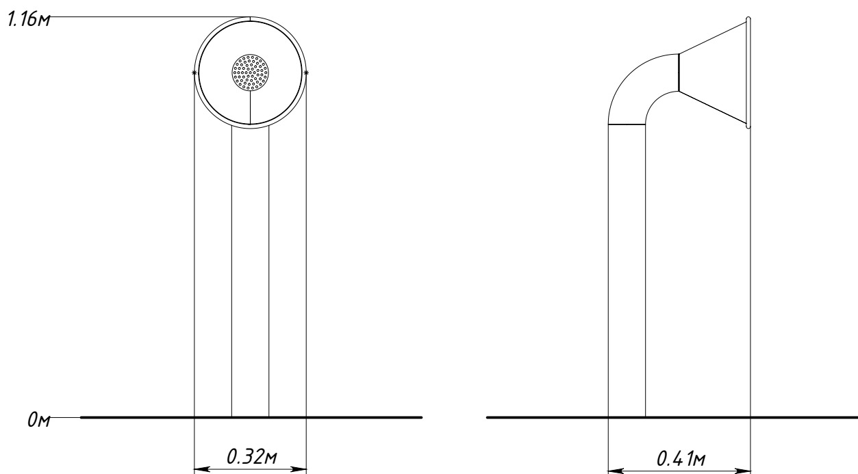
Рисунок 1 — Основные габаритные размеры
