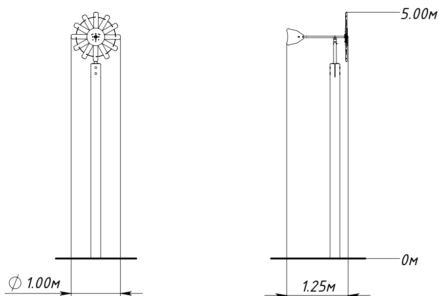
Рисунок 1 — Основные габаритные размеры
