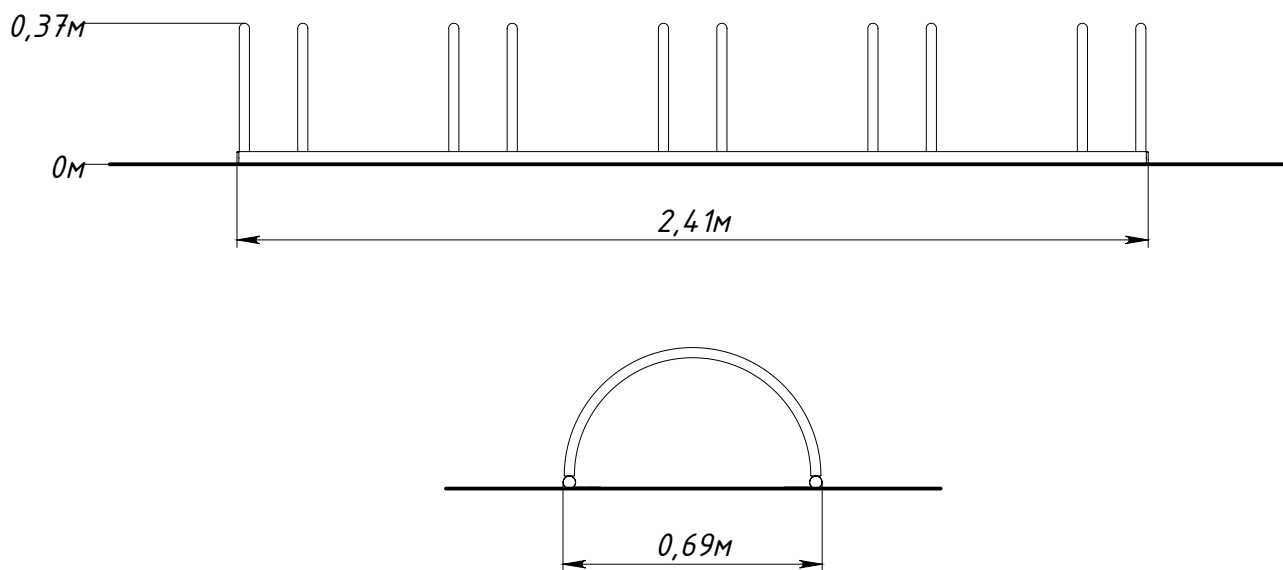
Рисунок 1 — Основные габаритные размеры
