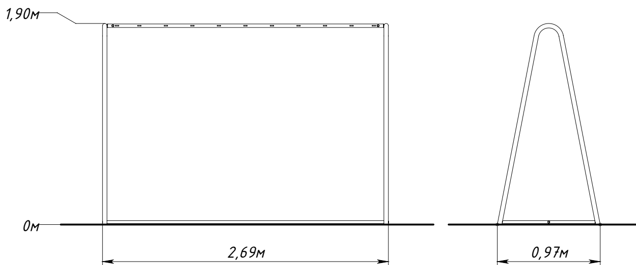
Рисунок 1 — Основные габаритные размеры
