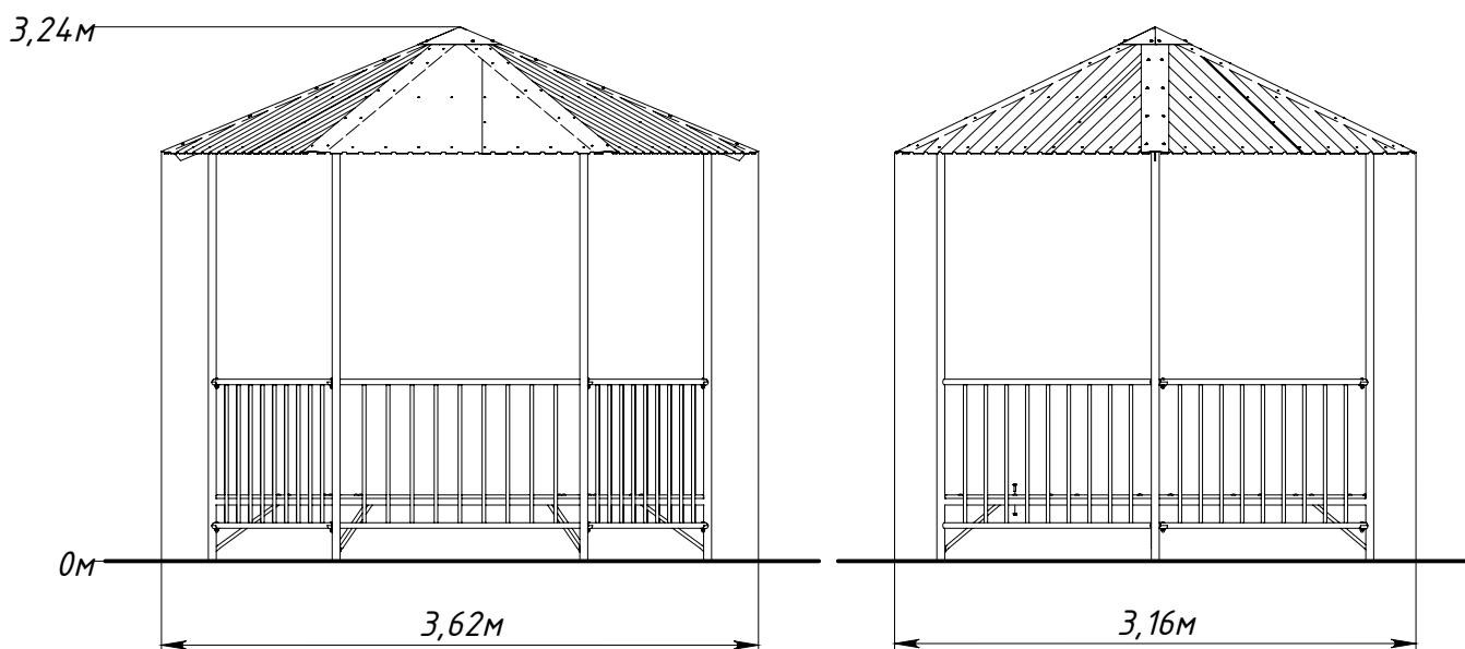
Рисунок 1 — Основные габаритные размеры
