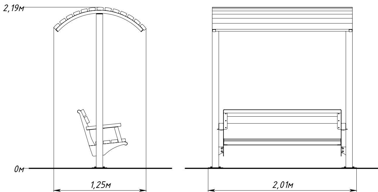
Рисунок 1 — Основные габаритные размеры
