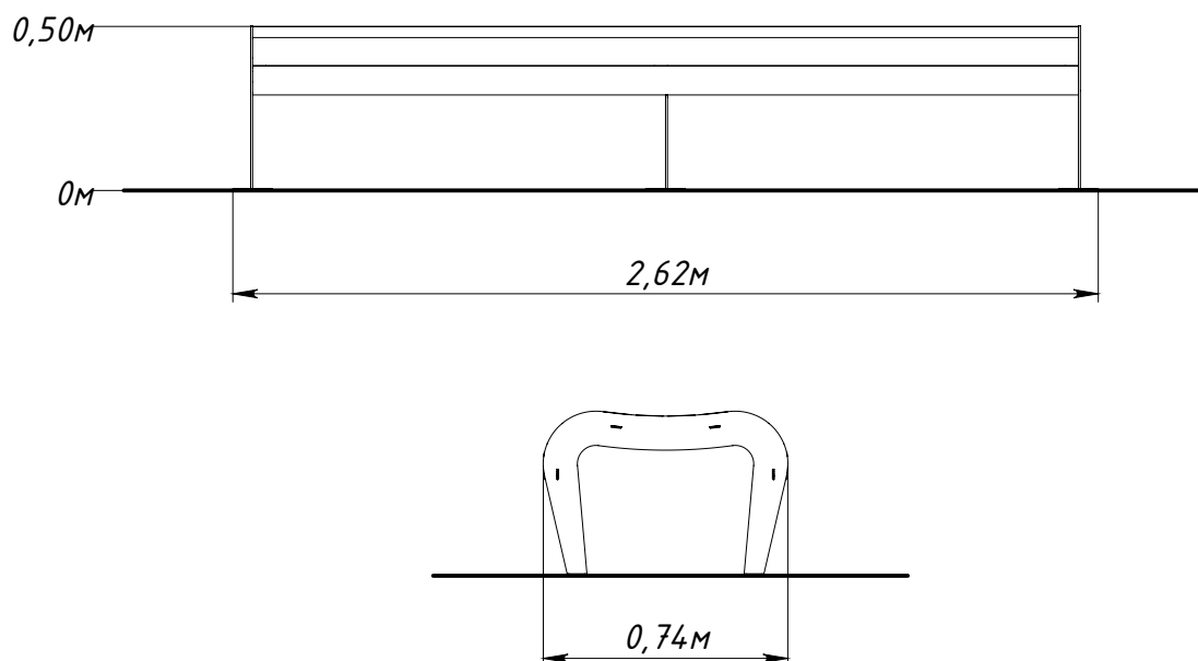
Рисунок 1 — Основные габаритные размеры
