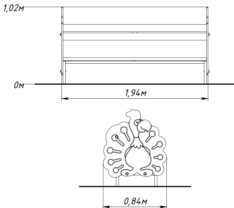
Рисунок 1 — Основные габаритные размеры
