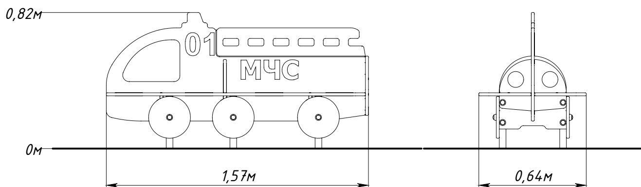
Рисунок 1 — Основные габаритные размеры
