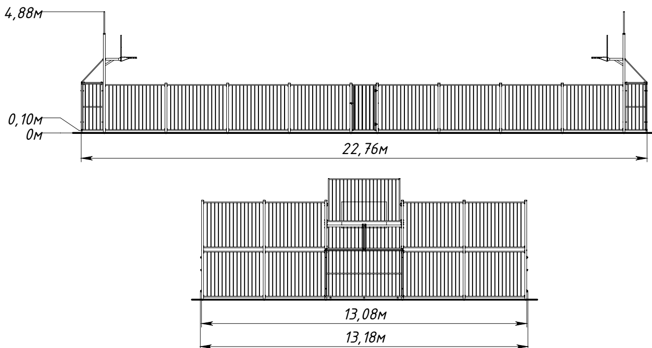
Рисунок 1 — Основные габаритные размеры
