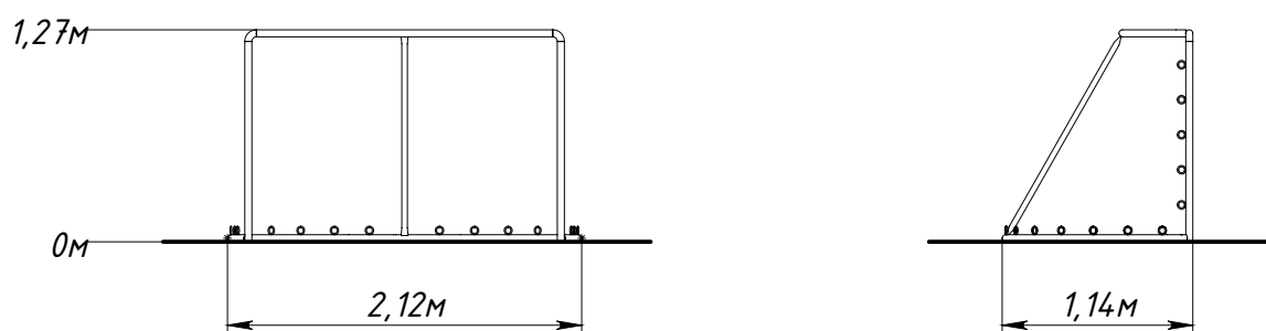
Рисунок 1 — Основные габаритные размеры
