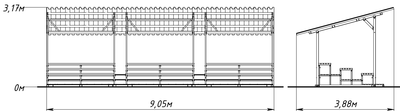
Рисунок 1 — Основные габаритные размеры
