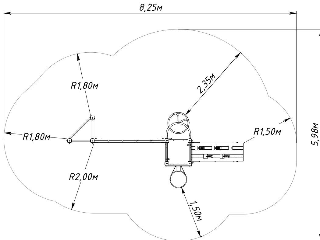
Рисунок 1 — Основные габаритные размеры
