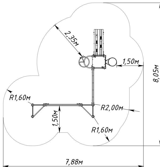
Рисунок 2 — Граница зоны приземления
