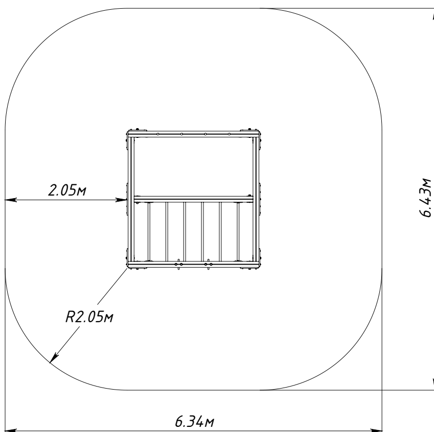
Рисунок 1 — Основные габаритные размеры
