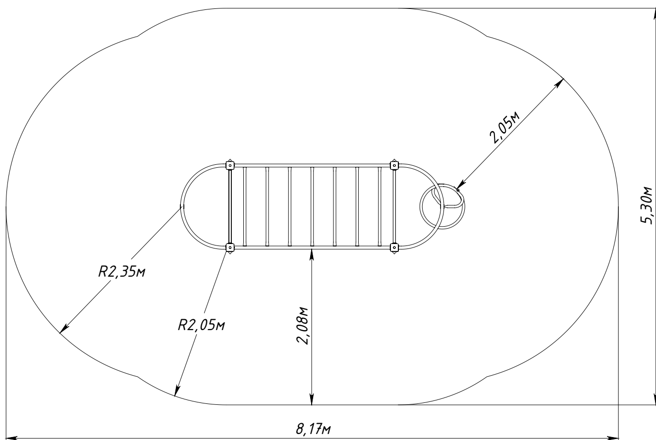
Рисунок 1 — Основные габаритные размеры
