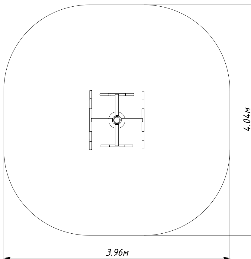
Рисунок 1 — Основные габаритные размеры
