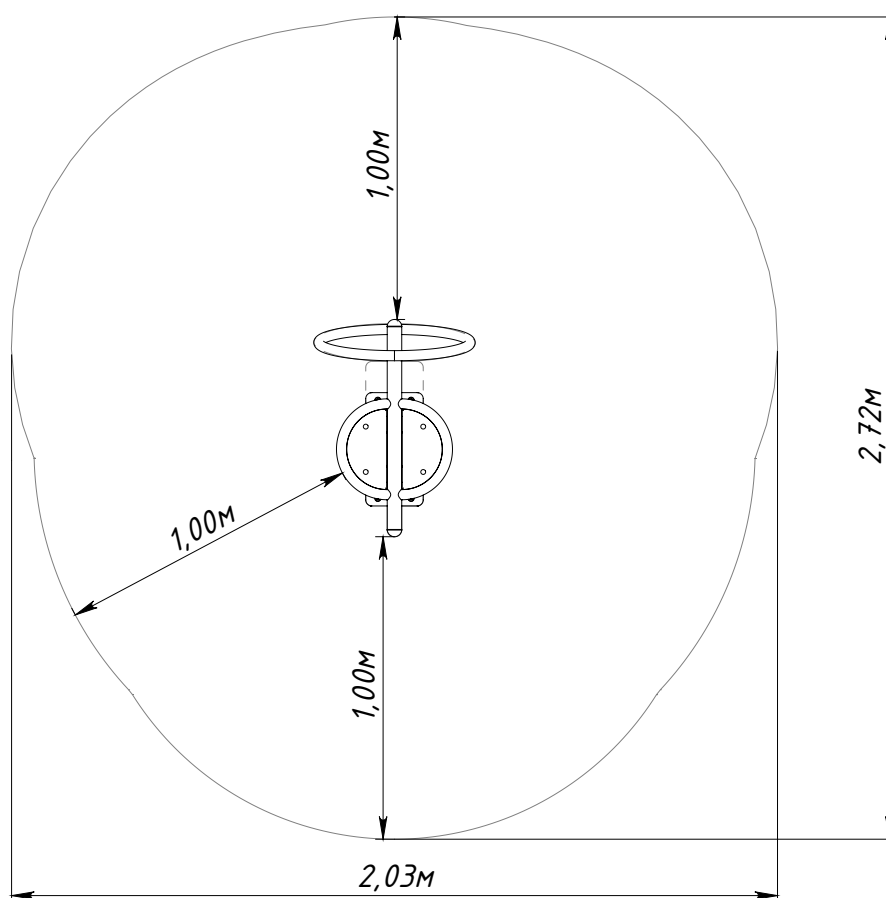
Рисунок 1 — Основные габаритные размеры
