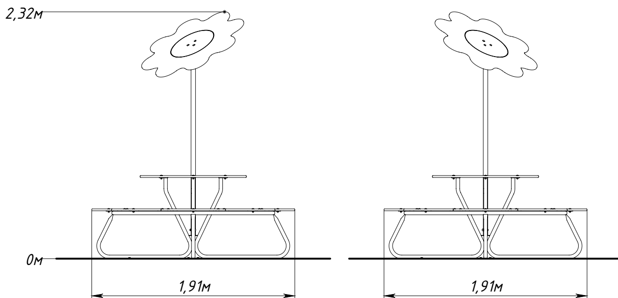
Рисунок 1 — Основные габаритные размеры
