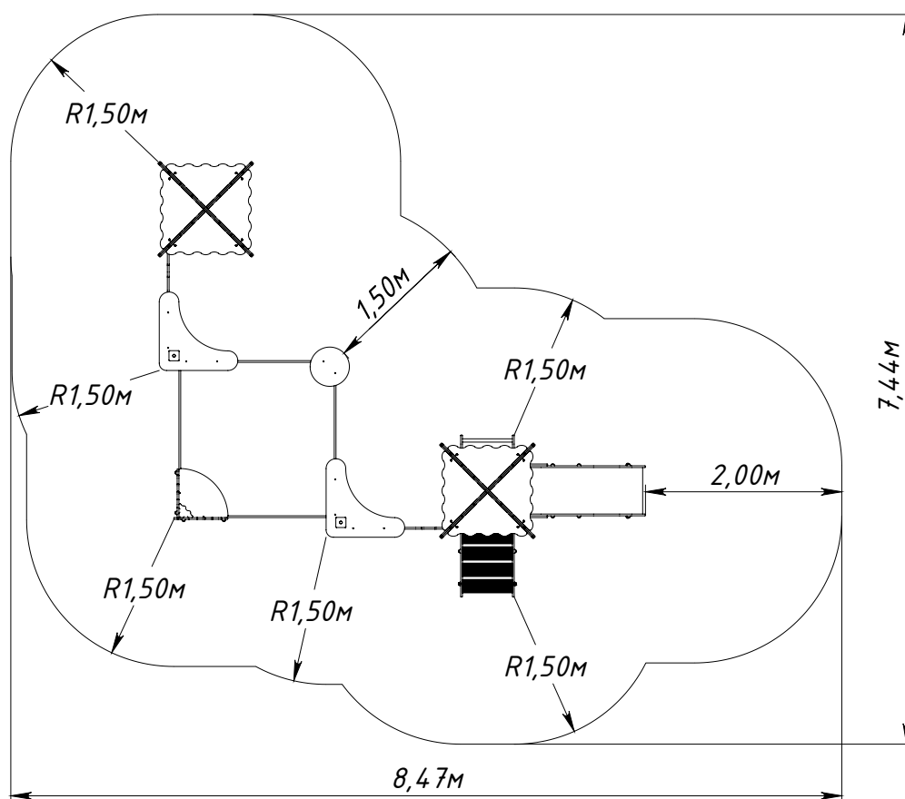
Рисунок 1 — Основные габаритные размеры
