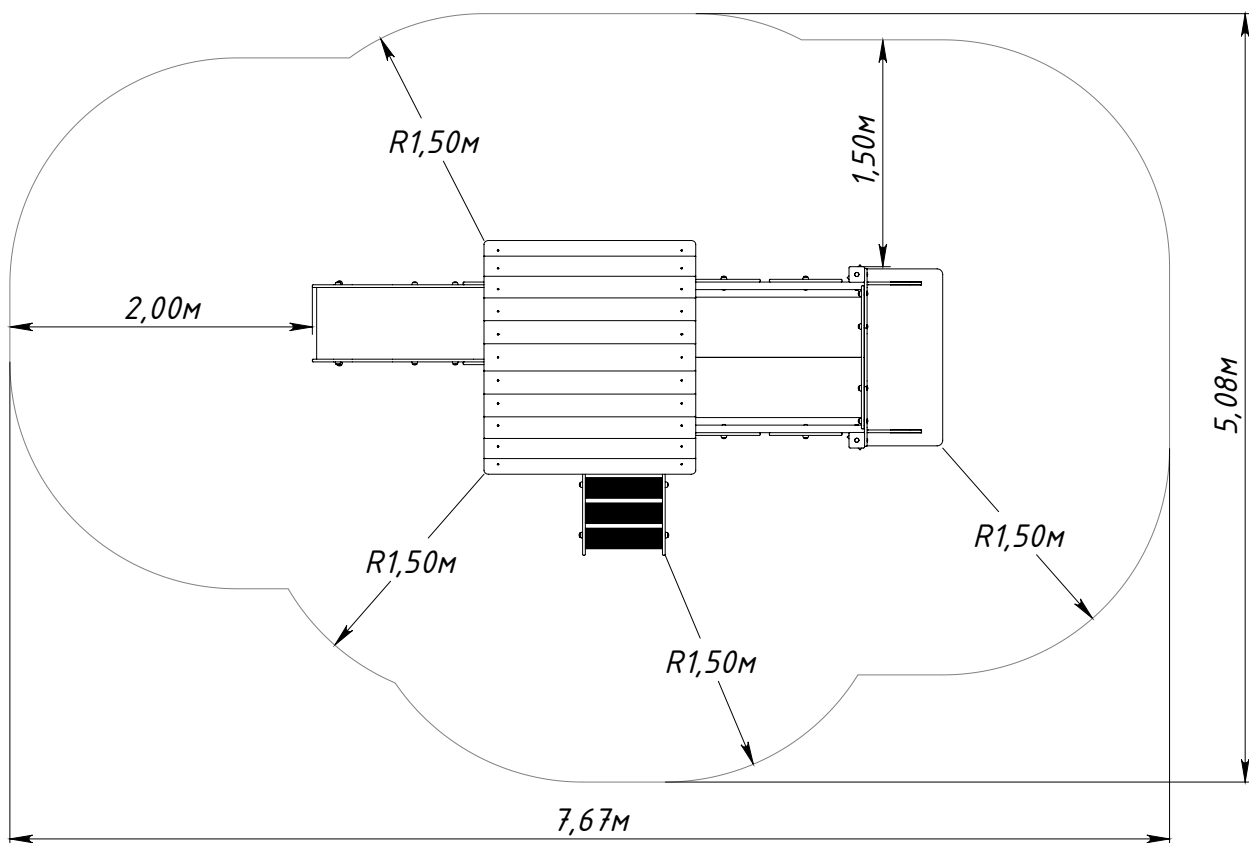
Рисунок 2 — Граница зоны приземления
