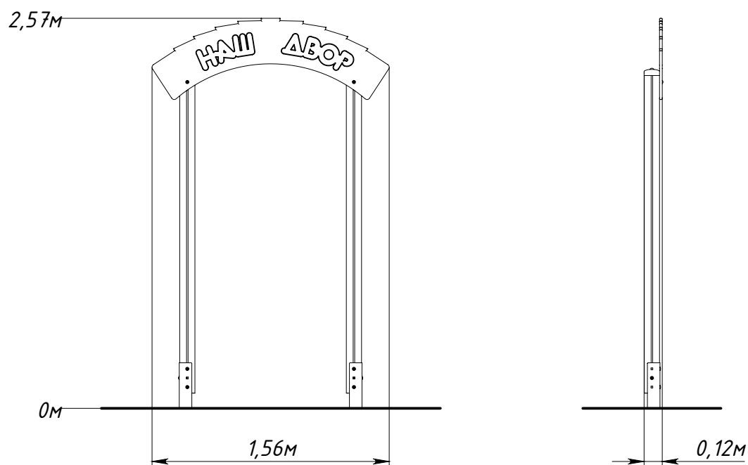
Рисунок 1 — Основные габаритные размеры
