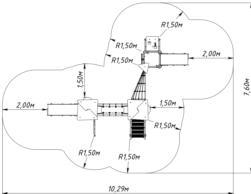
Рисунок 1 — Основные габаритные размеры
