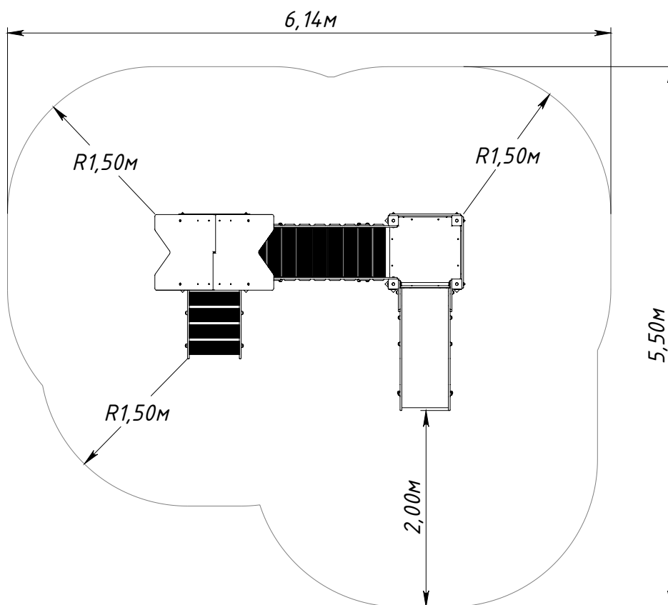
Рисунок 1 — Основные габаритные размеры
