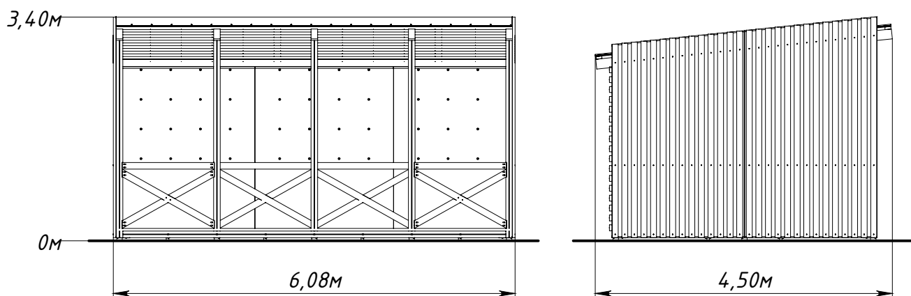
Рисунок 1 — Основные габаритные размеры
