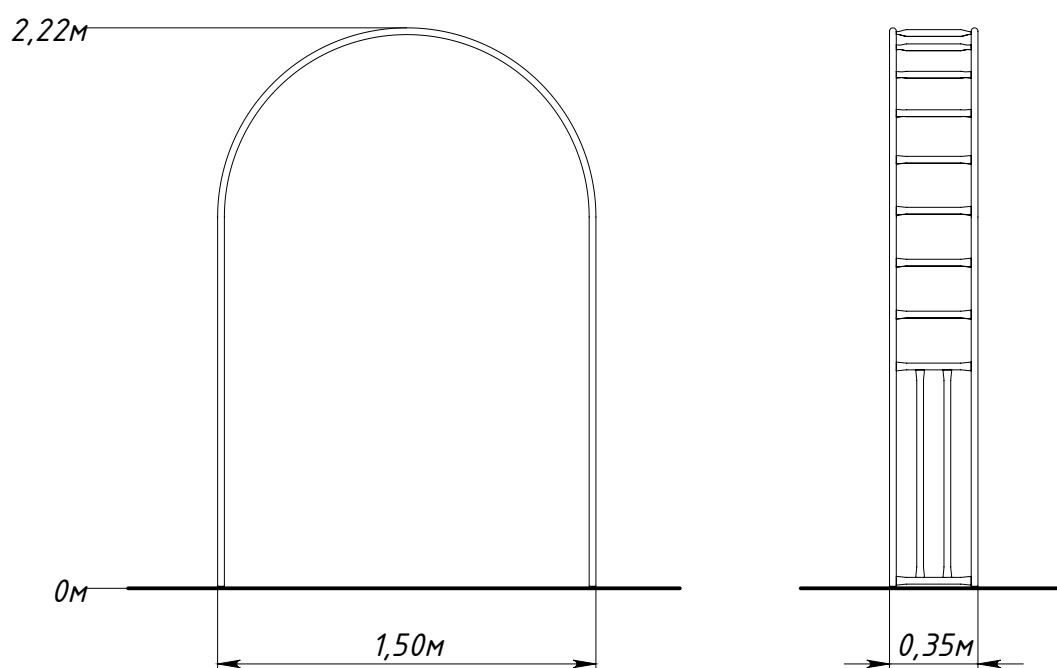
Рисунок 1 — Основные габаритные размеры
